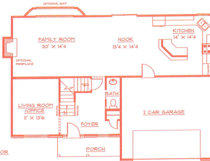
OPTIONAL FIREPLACE
